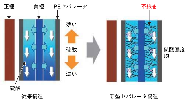
図1 従来構造と新型セパレータ構造における成層化現象
