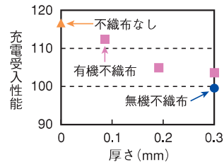
図2 新型セパレータ構造における種々不織布の充電受入性能への影響
